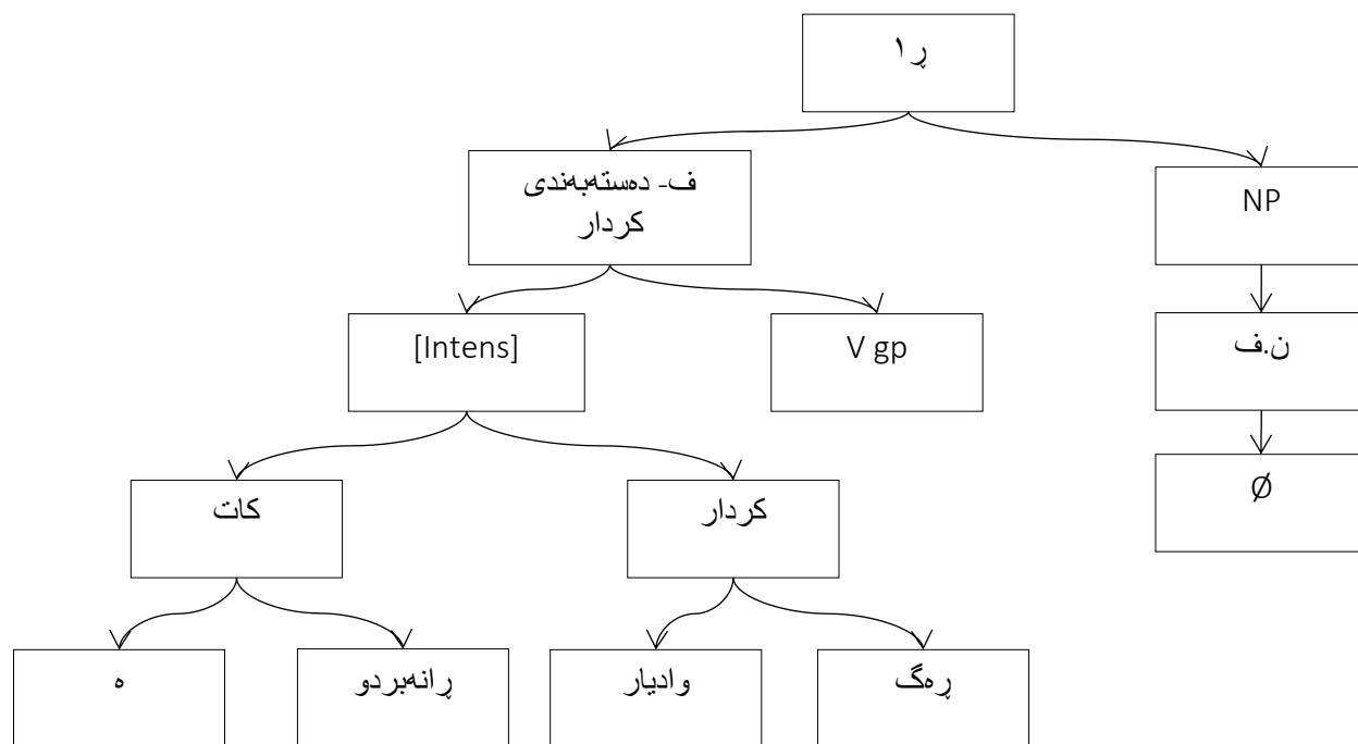
هێلکاری (٤): شیکردنهوهی درهختی بۆ رستهی (وا دیاره ئازاد نایهت).
