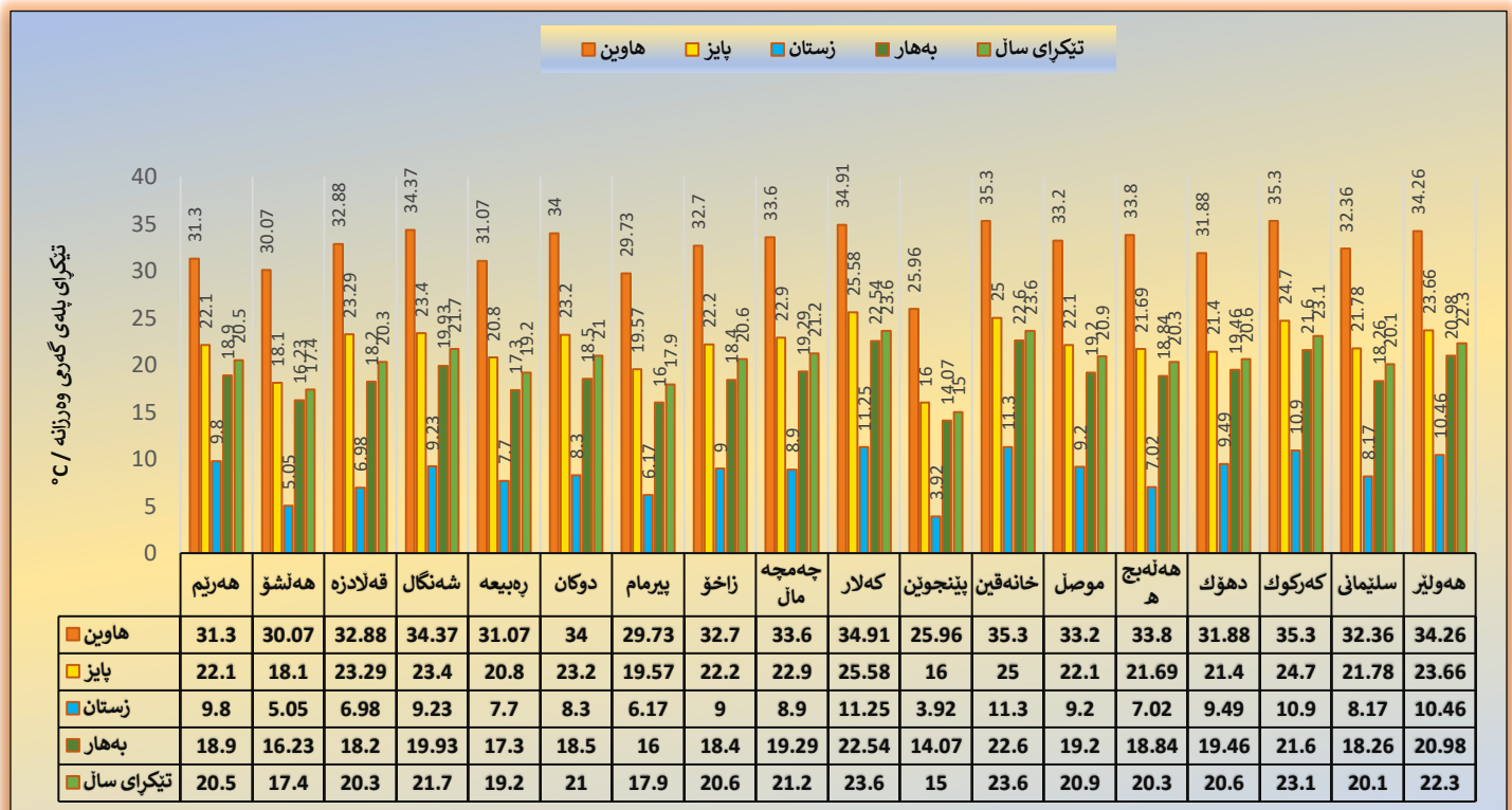
هیلکاری (2-2): تیکرای وه رزانه و سالانه ی پلهی گهرمی له ویستگه کانی ههریمی کوردستان له نیوان (2000-2021) C/ °. (2)
